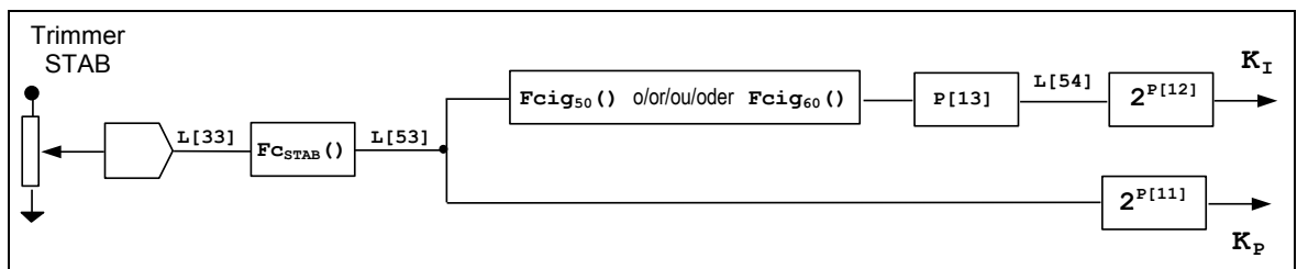
fig. 8a: schema delle elaborazioni numeriche dei guadagni proporzionale e integrale nel DER1 (standard) con trimmer STAB abilitato
