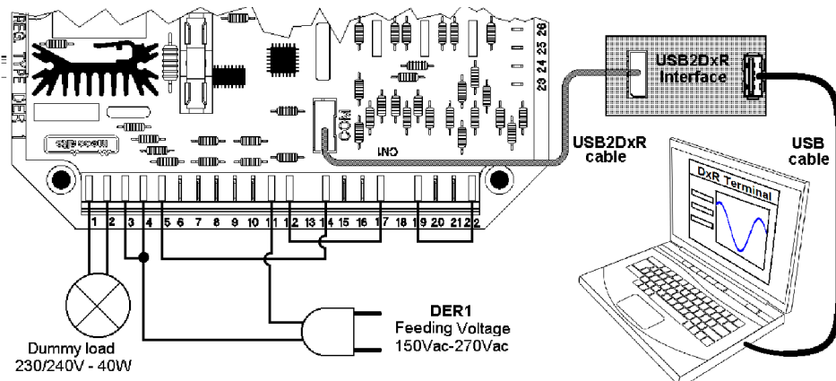
Fig. 12c: Alimentazione DER1 150-270Vac per test e impostazione
