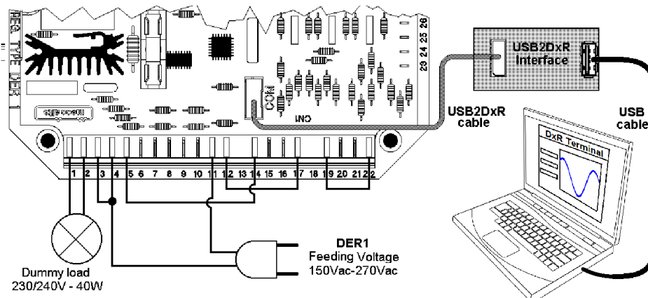
Fig. 12c: Alimentazione DER1 150-270Vac per test e impostazione
