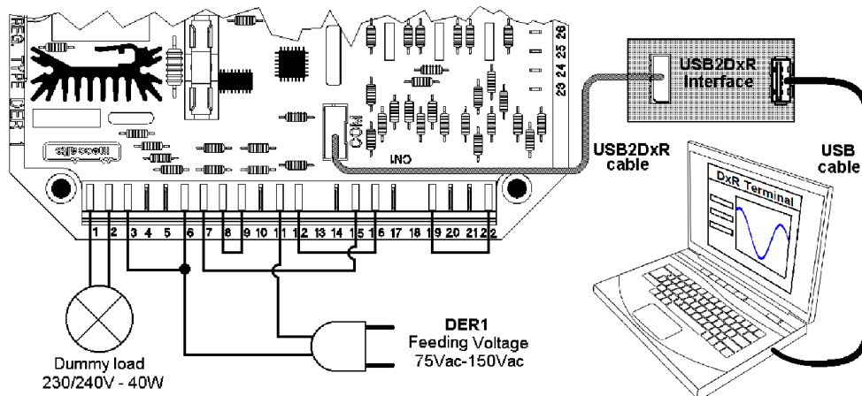
Fig. 12b: Alimentazione DER1 75-150Vac per test e impostazione
