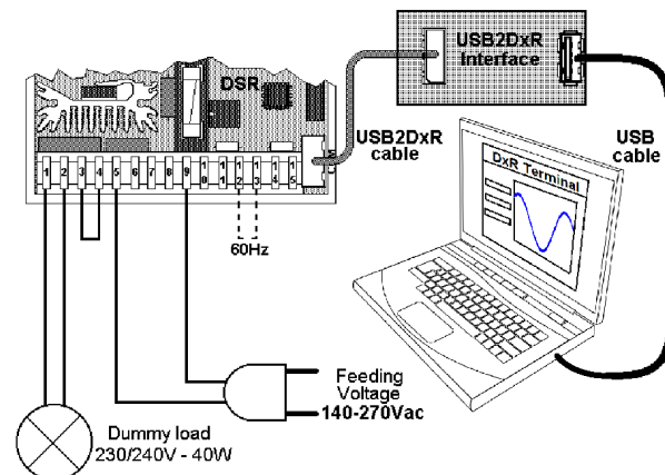
Fig. 11c: Alimentazione DSR 140-270Vac per test e impostazione
