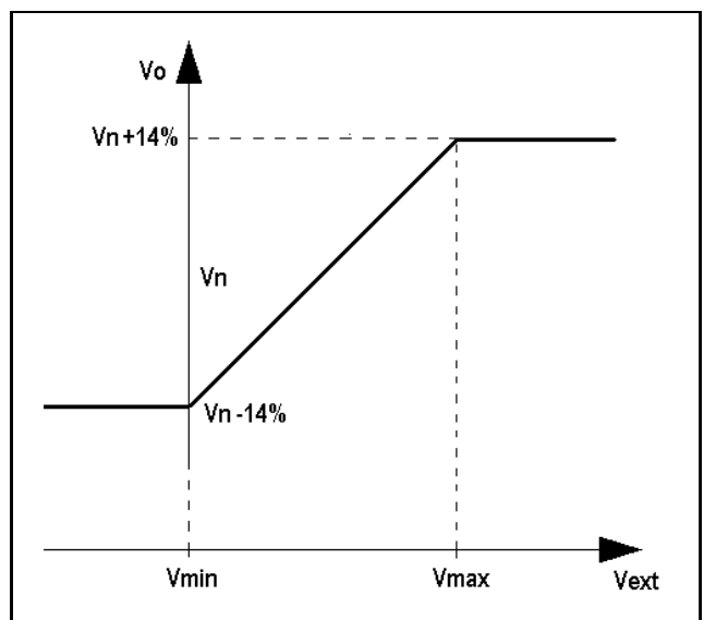
Figura 3b: con saturazione della tensione di uscita al raggiungimento dei limiti della tensione di ingresso
