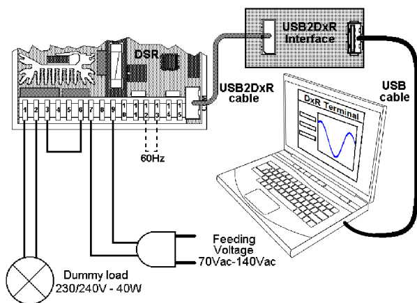
Fig. 11b: Alimentazione DSR 70-140Vac per test e impostazione
